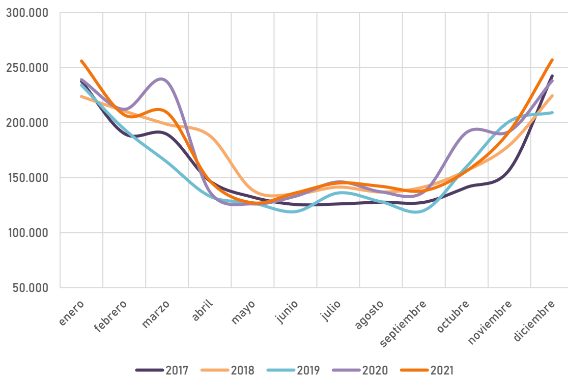
Gráfico 3: Demanda residencial mensual de Energía eléctrica en la provincia del Chaco para los años 2017-2021 (en MWh)
