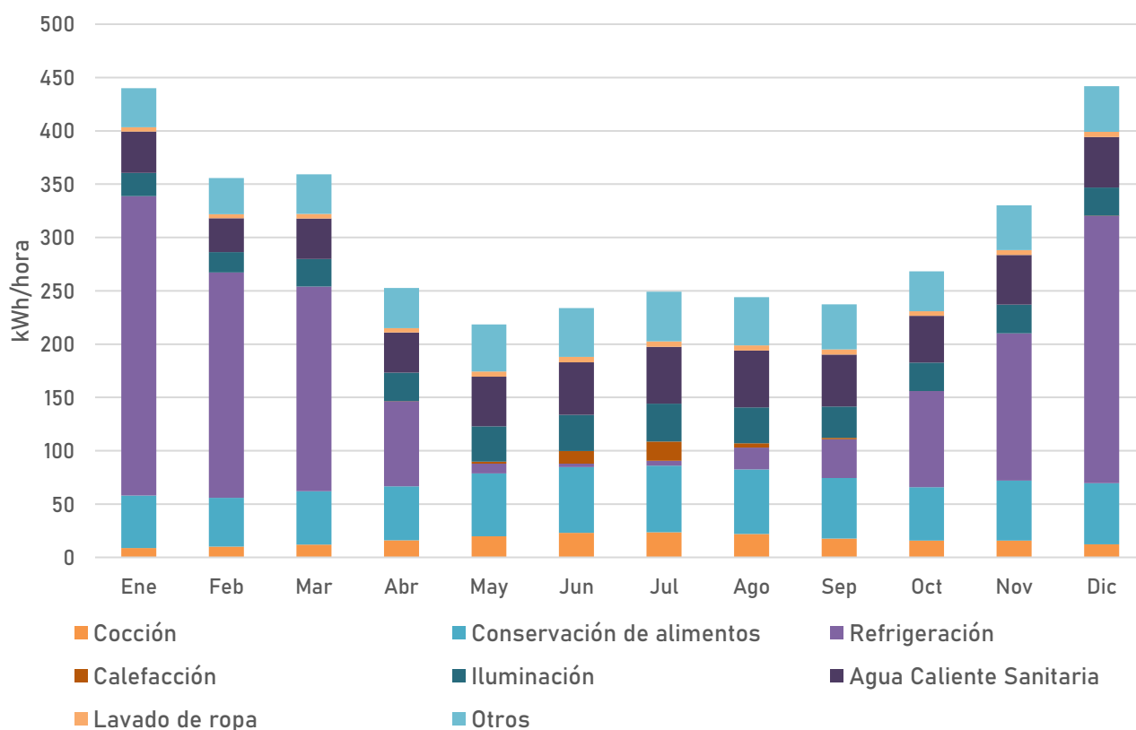
Gráfico 4: Distribución mensual de los usos de la energía de un hogar Chaqueño (año 2021)
